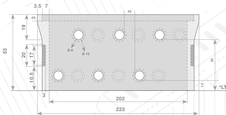
* linea di terra * ligne de terre
