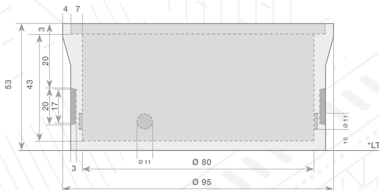
Vista frontale in sezione Vue avant en coupe
