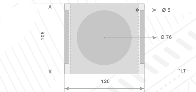
Vista frontale in sezione Vue avant en coupe
