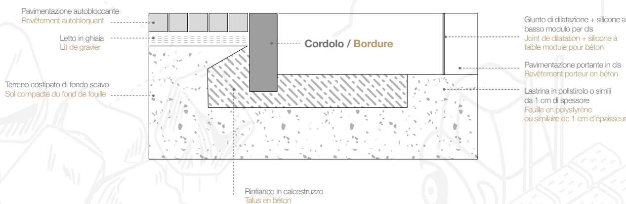
Caso con autobloccante e cordolo a bordo strada Cas avec pavé autobloquant et bordure de trottoir
