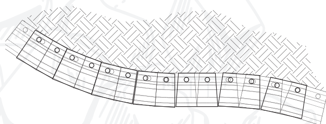
Schema di posa visto dall'alto Schéma de pose vu de dessus
