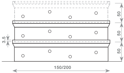
Esempio di posizionamento in batteria Exemple de positionnement de la batterie
