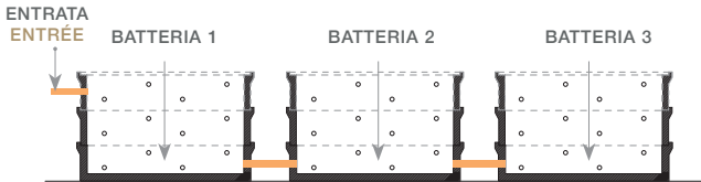
Esempio di posizionamento in batteria Exemple de positionnement de la batterie
